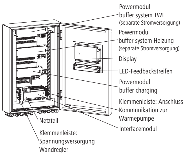
Abb. 1: Komponenten Wandregler
