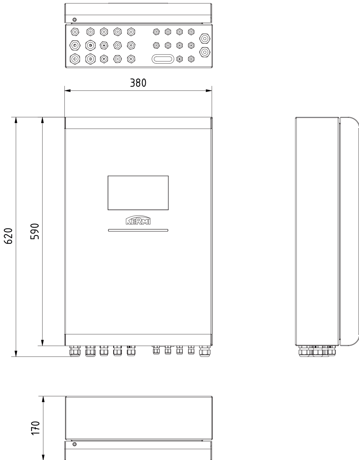
Abb. 7: Abmessungen Wandregler
