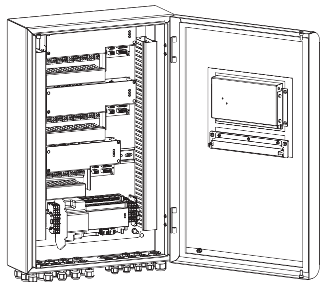
Abb. 4: Geöffneter Regler
