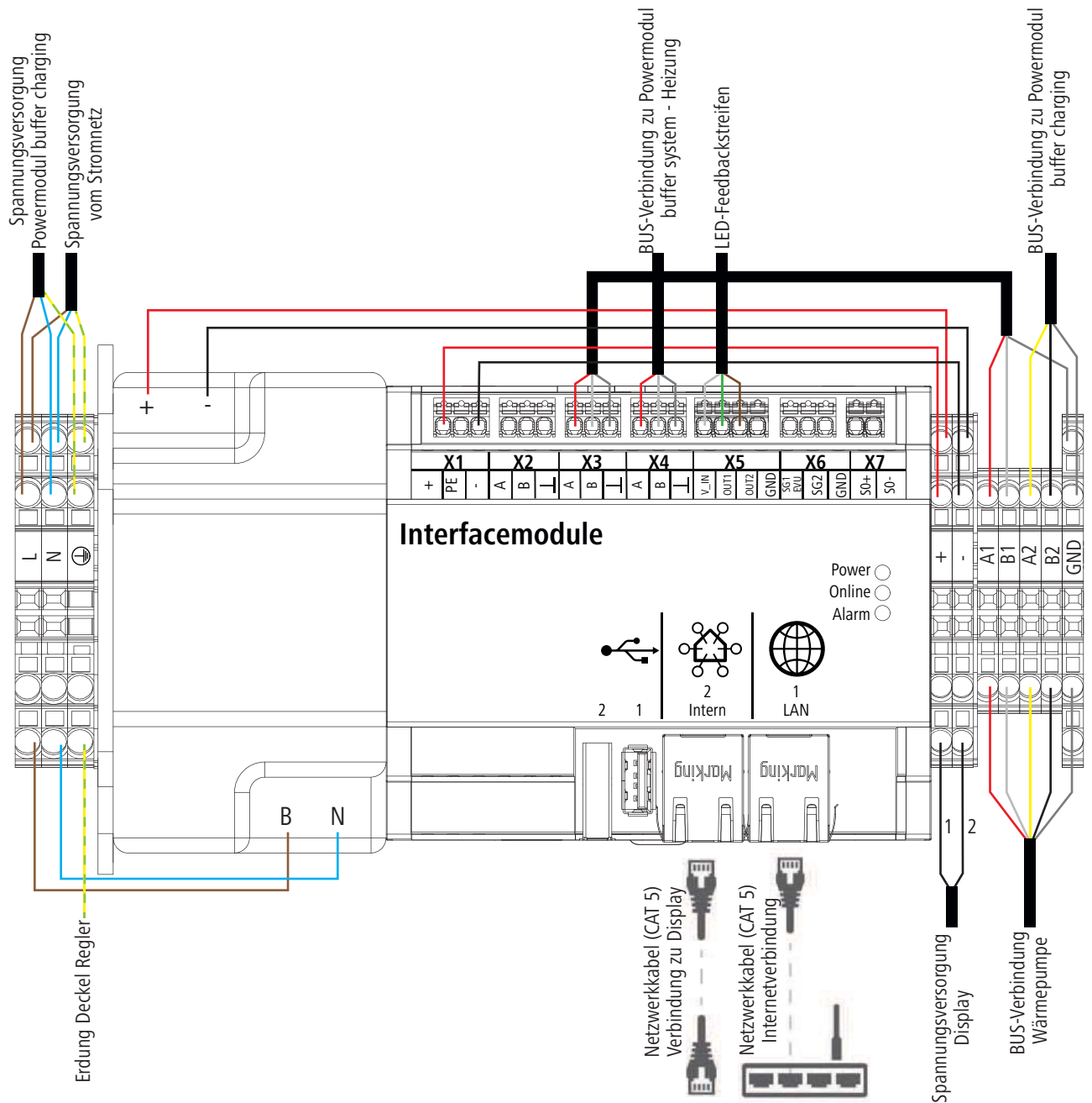
Abb. 10: Klemmenplan Klemmenleiste mit Interfacemodul
